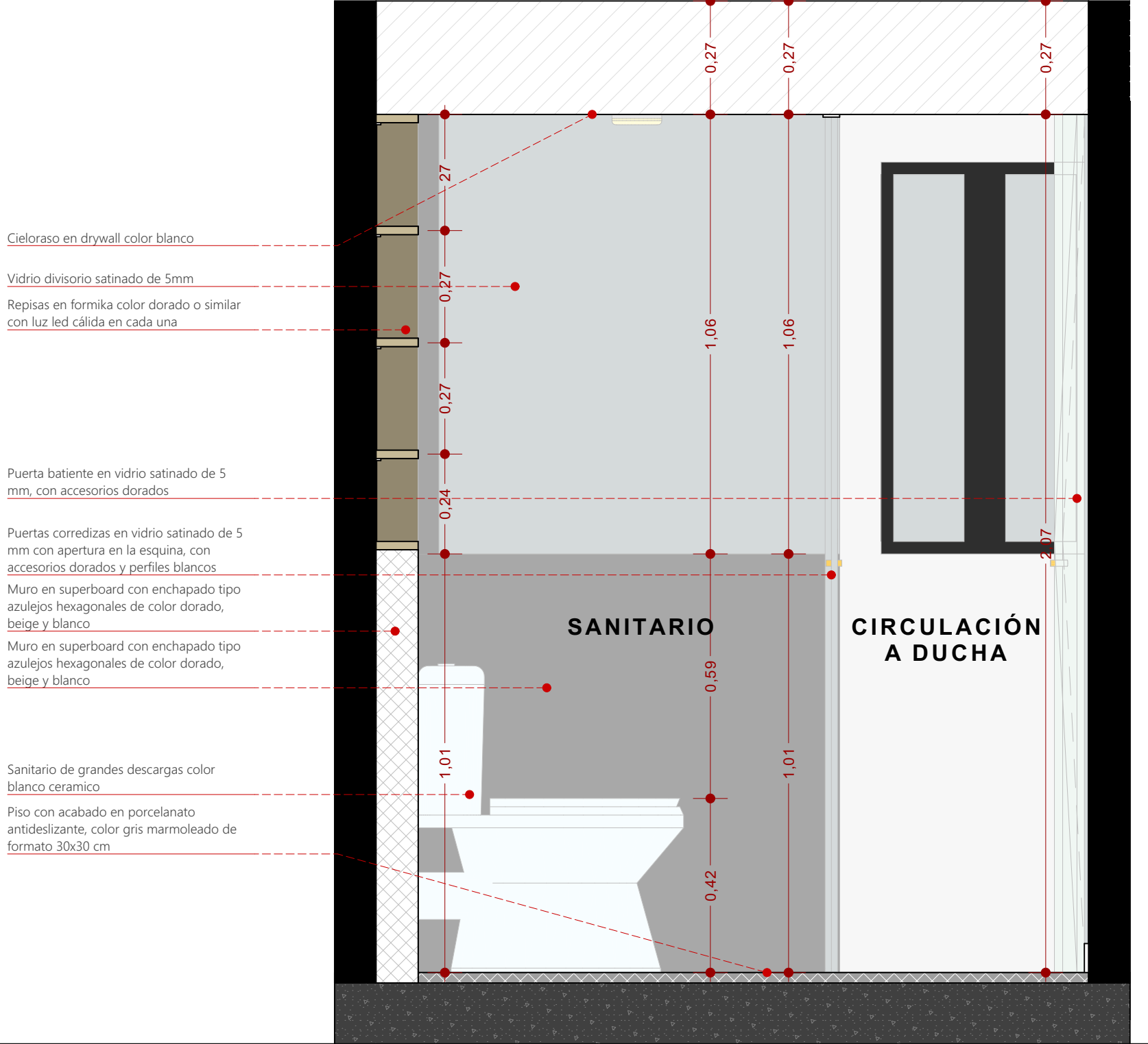
CORTE B-B'
