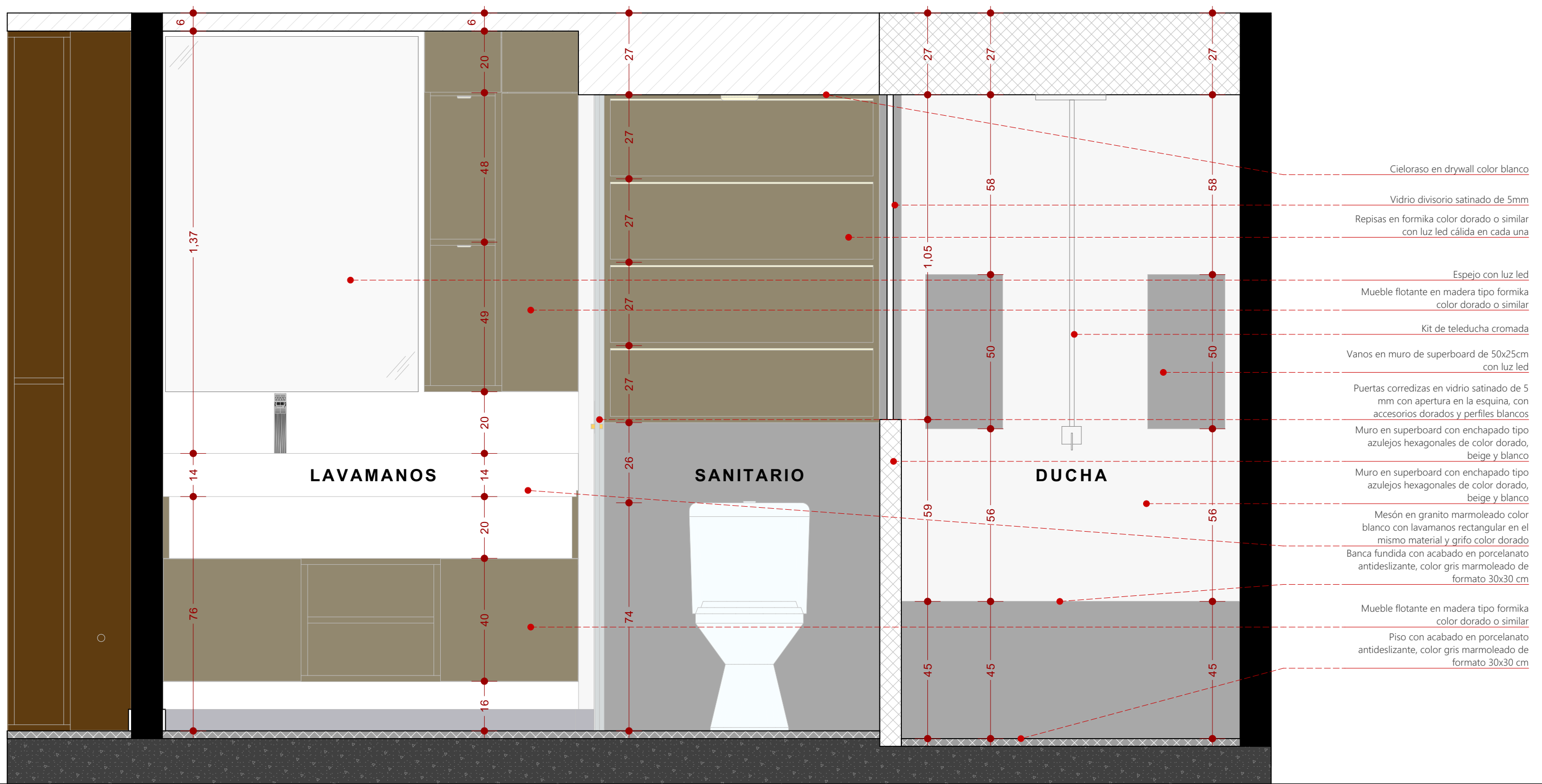
CORTE A-A'
